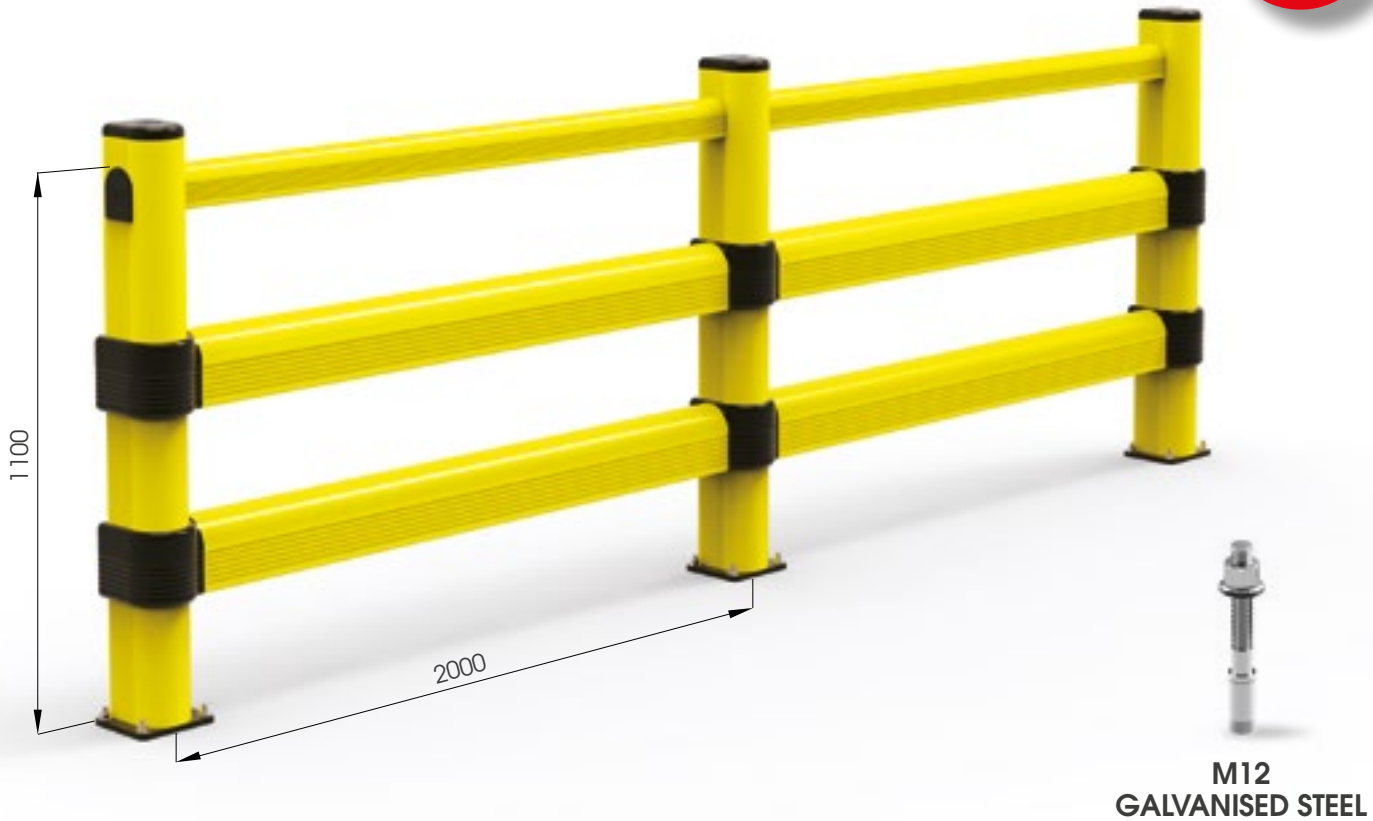
LINK 150/2
