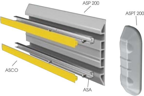
ASP 200
